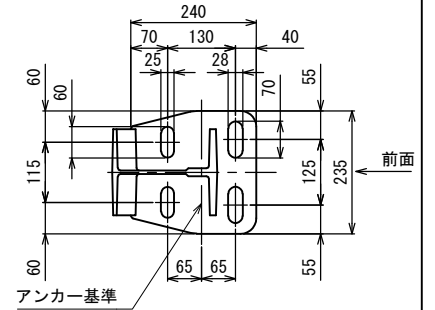
A-A断面 (アンカー部詳細)
